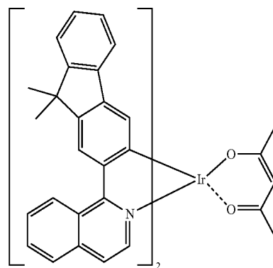
Ir(fliq) 2 (acac)
