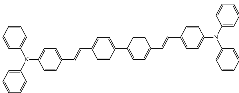
DPVBi DPAVB
