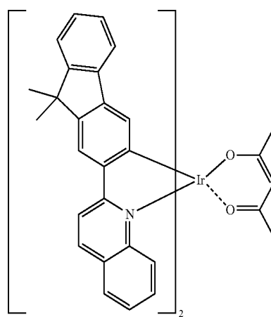
Ir(flq) 2 (acac)
