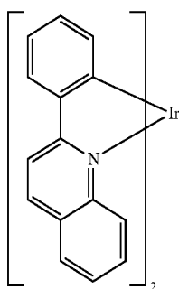
Ir(2-phq) 3
